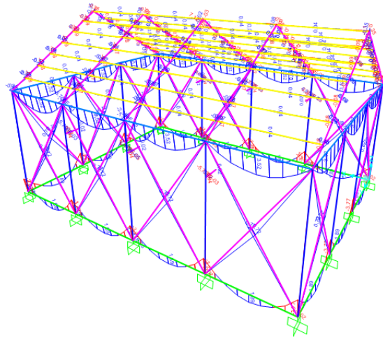
Gambar 4. Perilaku momen hasil analisis
