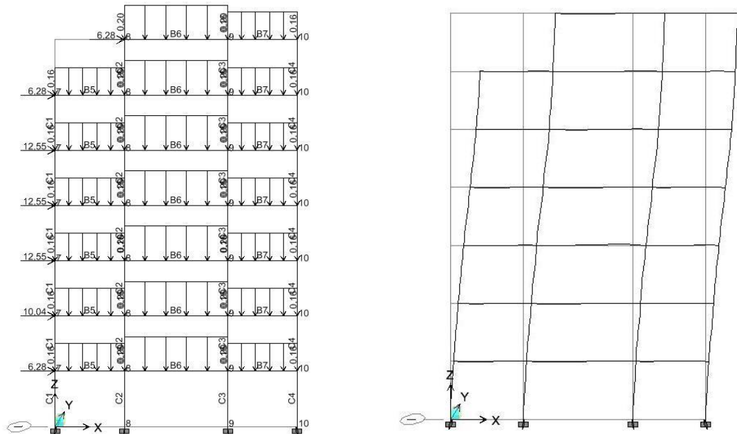
Gambar 2. Model struktur portal (kiri) dan deformasinya (kanan) pada ETABS
