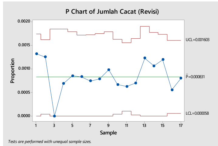
Gambar 4. Perbaikan Control p -Chart Komponen Foxing Periode Juli 2020
