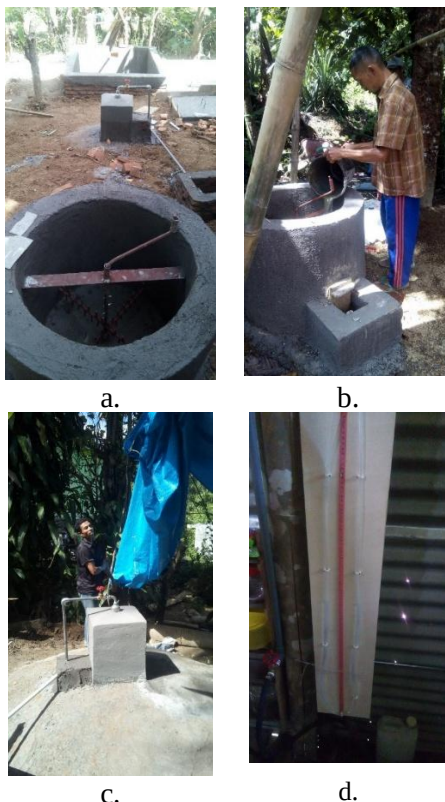
Gambar 1 a. bak pengadukan kotoran sapi, b. proses pencampuran kotoran sapi dengan air, c. tangki digester kapasitas 4 m 3 , d. pengukuran tekanan gas menggunakan manometer sederhana.
