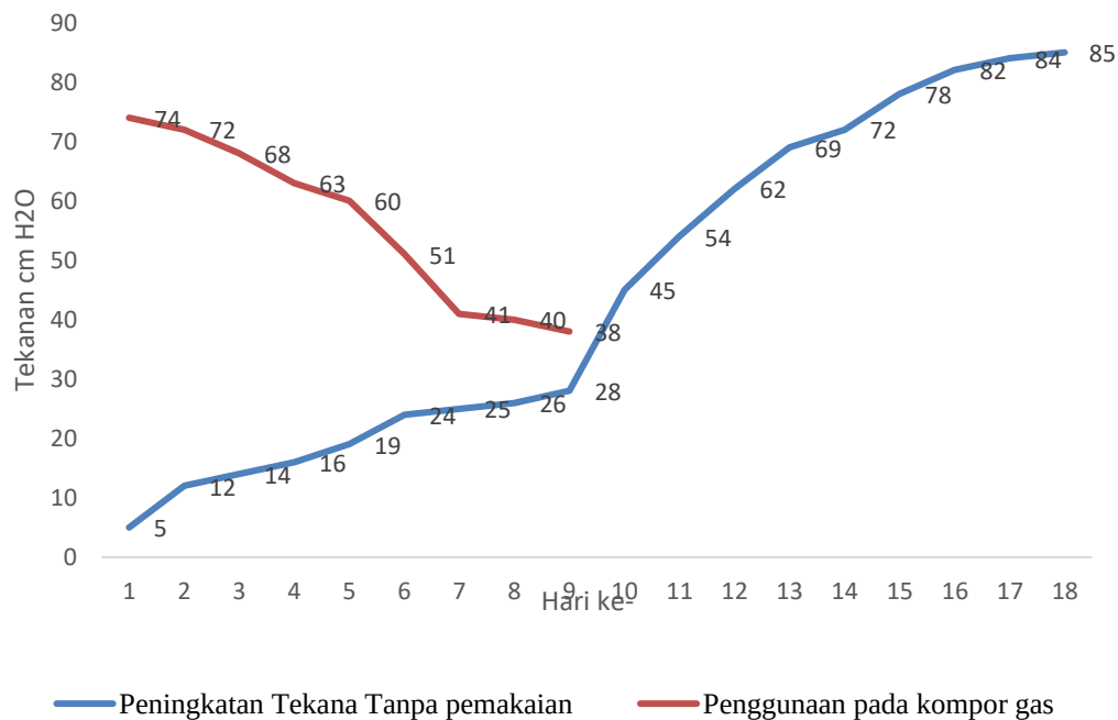
Gambar 3. Tekanan biogas pada digester
