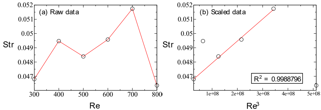
Gambar 3. Plot frekuensi Str terhadap bilangan Re (a) raw data (b) scaled data
