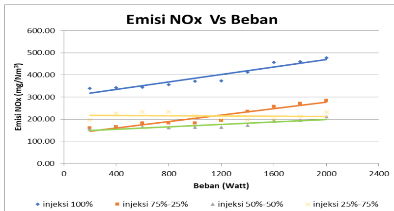
Gambar 7. Grafik emisi NOx terhadap beban
