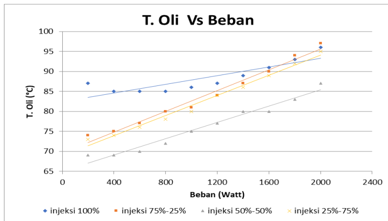
Gambar 4. Grafik temperatur engine terhadap beban
