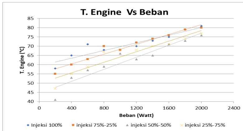
Gambar 4. Grafik temperatur engine terhadap beban
