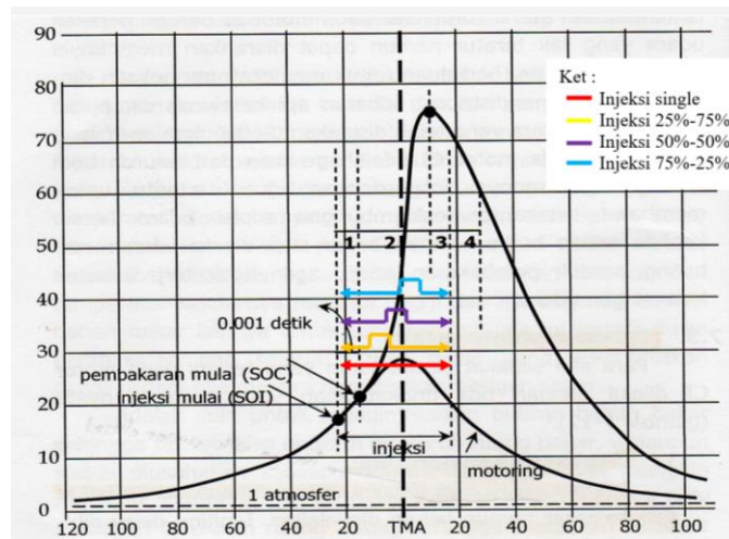
Gambar 1. Grafik P-θ skema injeksi bertingkat
