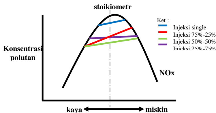
Gambar 8. Grafik tipikal polutan NOx
