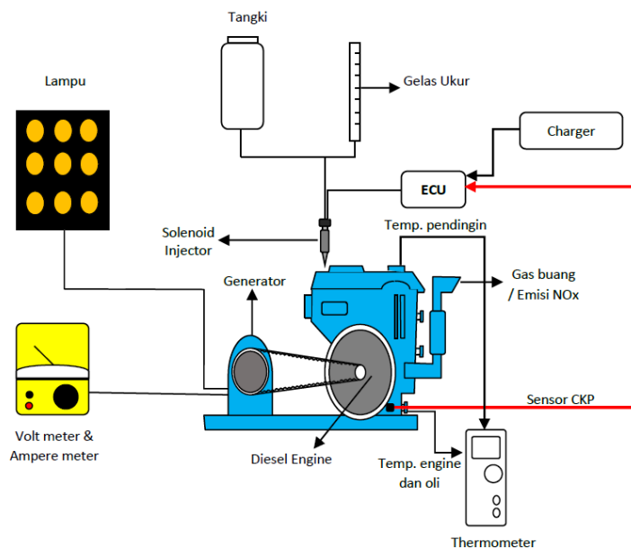
Gambar 2. Skema alat ukur penelitian
