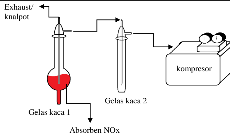
Gambar 3. skema alat ukur emisi NOx
