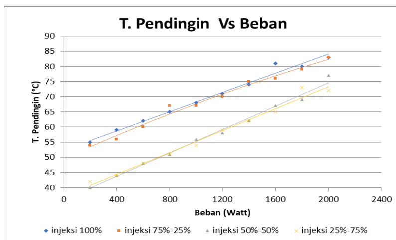
Gambar 6. Grafik temperatur pendingin terhadap beban
