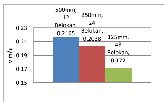
Gambar 11. Grafik Hubungan antara panjang tube setelah belokan dan jumlah belokan dengan kecepatan aliran
