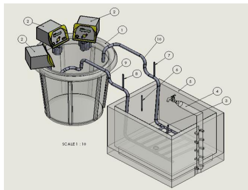
Gambar 1. Sketmatik peralatan penelitian
