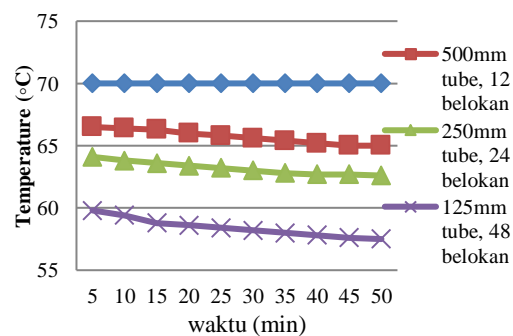
Gambar 7. Grafik Perbandingan Data Temperatur terhadap Waktu pada suhu inlet 70°C untuk Ketiga Jenis Variasi HE.
