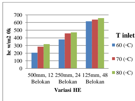
Gambar 10. Grafik Hubungan antara panjang tube setelah belokan dan jumlah belokan dengan nilai hc
