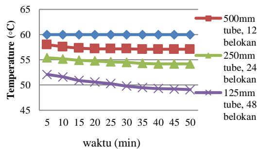
Gambar 6. Grafik Perbandingan Data Temperatur terhadap Waktu pada suhu inlet 60°C untuk Ketiga Jenis Variasi HE.
