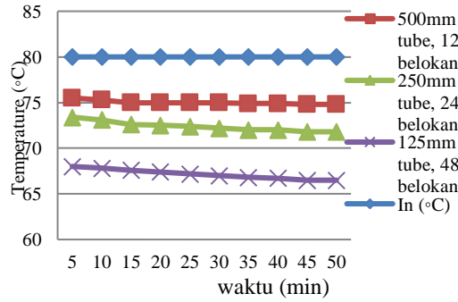
Gambar 8. Grafik Perbandingan Data Temperatur terhadap Waktu pada suhu inlet 80°C untuk Ketiga Jenis Variasi HE.
