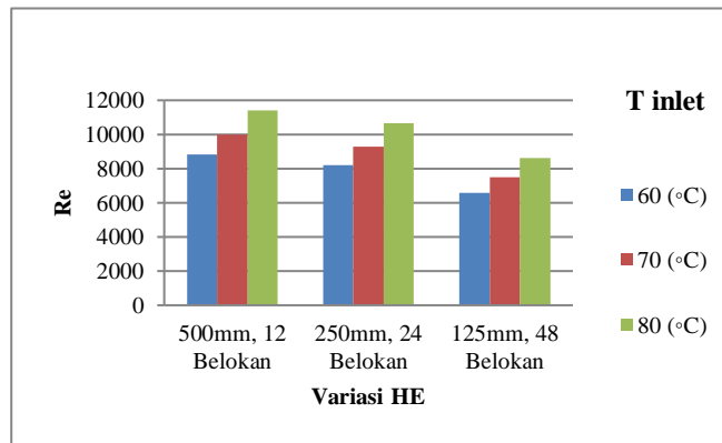
Gambar 9. Grafik Hubungan antara panjang tube setelah belokan dan jumlah belokan dengan nilai Re
