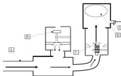
Gambar 9. Prinsip kerja pompa hidram.
